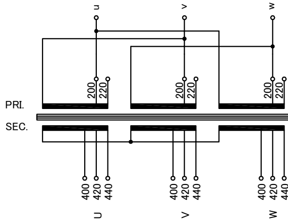
回路図
